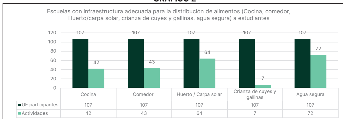
GRÁFICO 2
