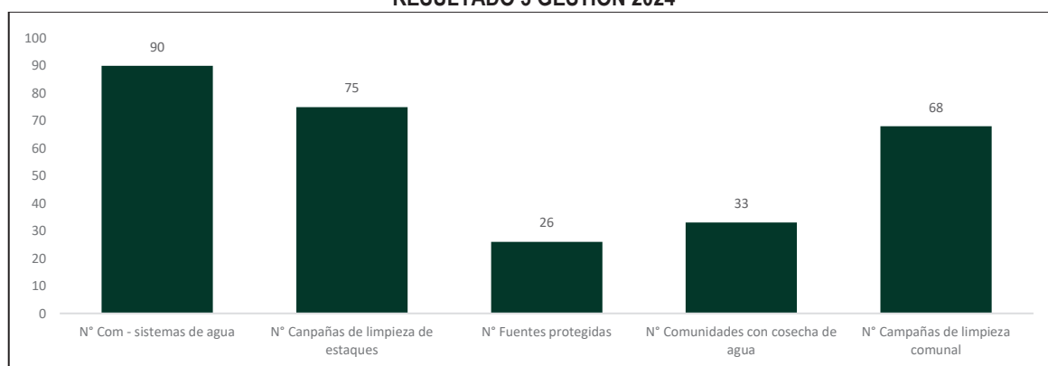
GRÁFICO 2 RESULTADO 3 GESTIÓN 2024
