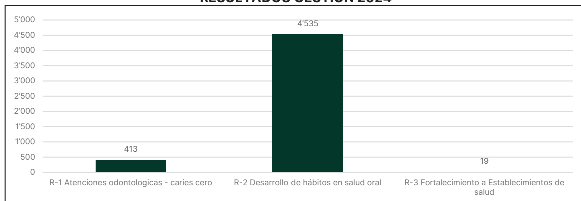
GRÁFICO 1 RESULTADOS GESTIÓN 2024
